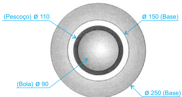
PLANTA BAIXA
